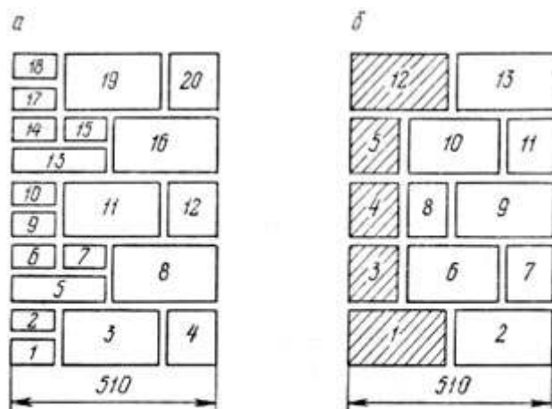
Рис. 8.30. Последовательность кладки с облицовкой: а — лицевым кирпичом; б — лицевым камнем (цифрами обозначена последовательность укладки кирпича и камней)
