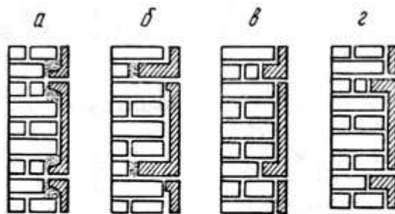
Рис. 8.31. Способы крепления плит с кладкой стен:
