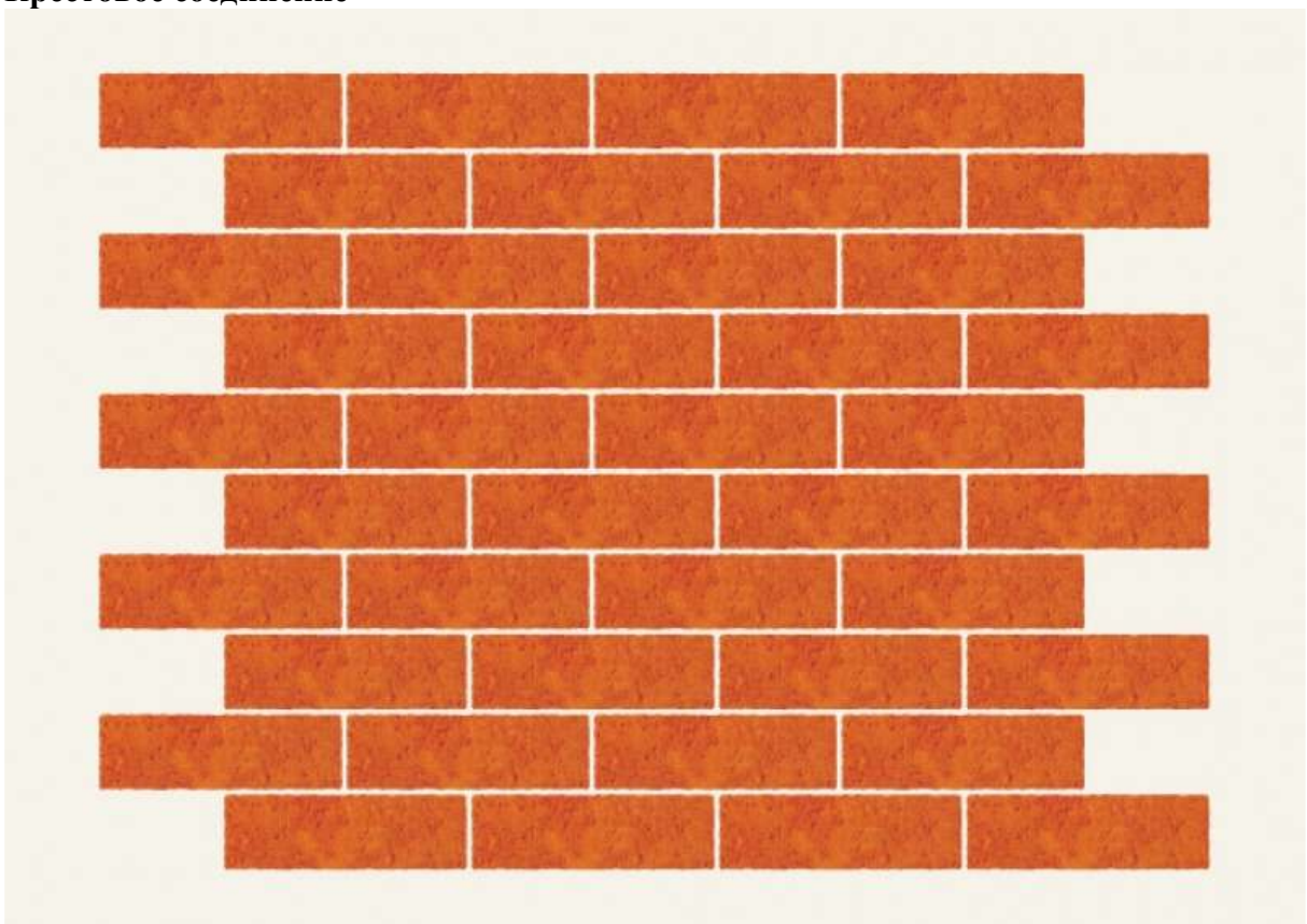
Рядовое соединение с 1/2 кирпича
