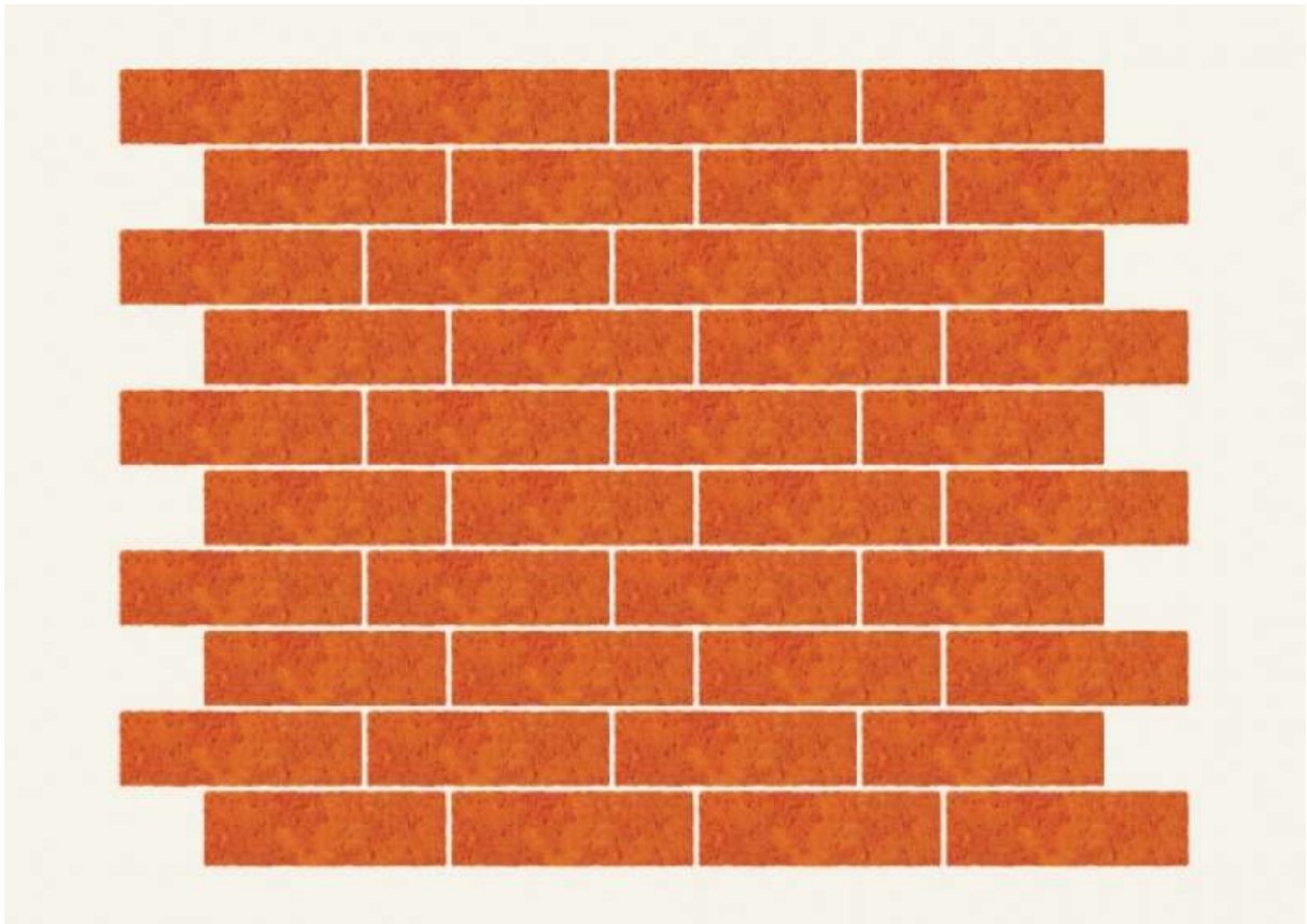
Рядовое соединение с 1/3 кирпича
